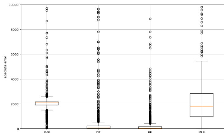
شکل ۸- مقایسه خطای مطلق مدل
